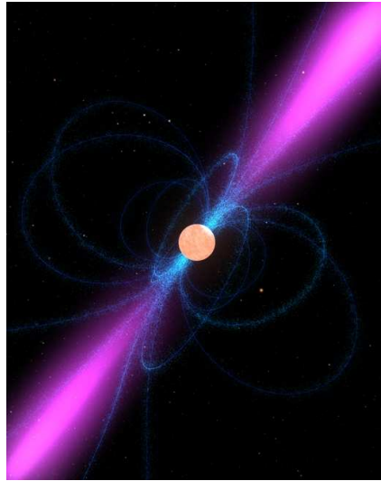
5.3. ábra. Pulzár illusztrációja. A neutroncsillagot tengelyszimmetrikus magnetoszférv teszi körül. Az elektromágneses sugárzás a mágneses tér poláris tartományából tör elő. [Forrás: http://www.nasaimages.org/ ]
