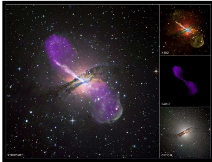
5.13. ábra. A Centaurus A aktív galaxis, valamint a galaxis síkjára közel merőleges nyalábok. A kép az optikai-, röntgen- és rádiótartományokban készült felvételek (hamis színekkel ábrázolt) szuperpozíciójaként állt elő. [Forrás: http://www.nasaimages.org/ ]
